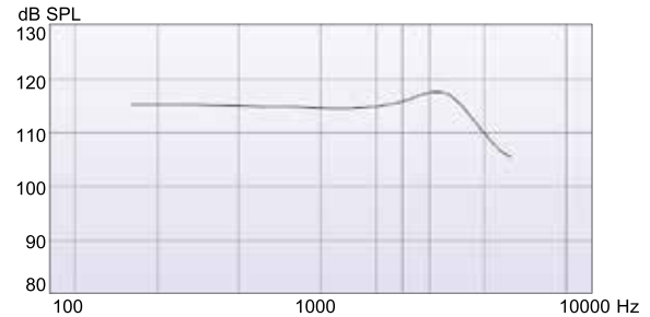
最大出力音圧 (入力音圧 90dB SPL)
